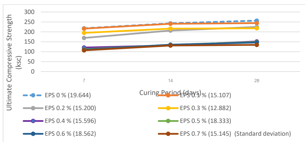
ภาพที่ 2 การเปรียบเทียบค่ากำลังอัดในแต่ละสัปดาห์ของอิฐอิฐโฟมในคอนกรีตตัวอย่างที่อายุบ่ม 7 14 28 วัน
